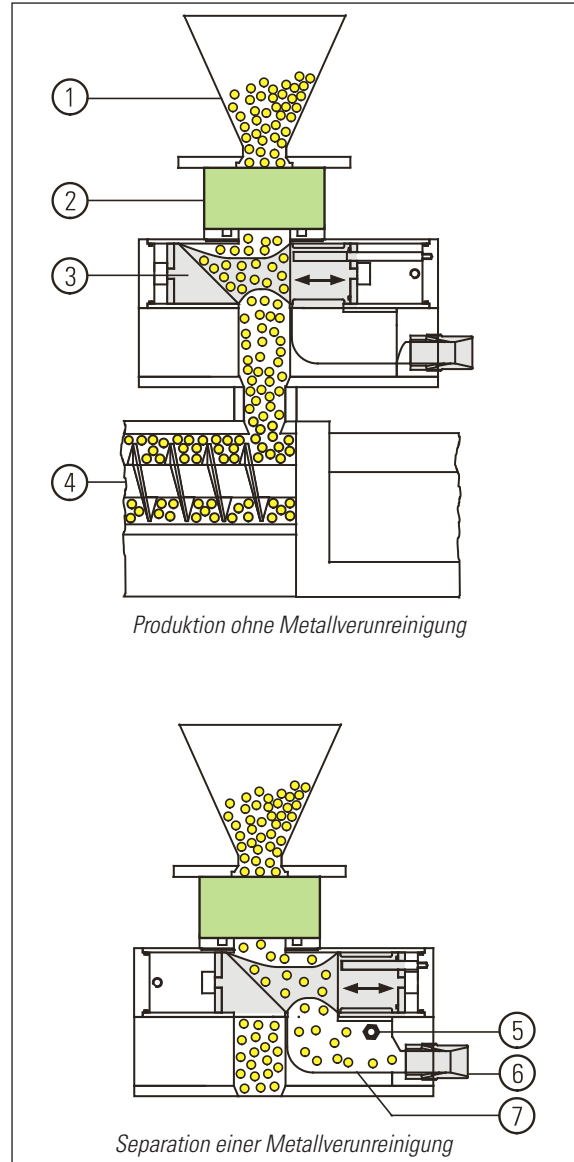
Metall-Separator PROTECTOR angebaut am Materialeinzug einer Spritzgießmaschine
