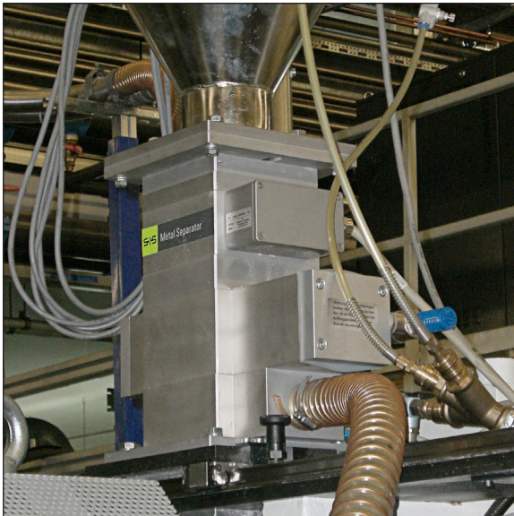
Metall-Separator PROTECTOR angebaut am Materialeinzug einer Spritzgießmaschine
